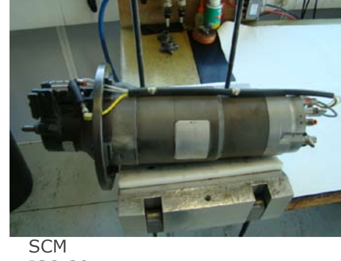
HSD ES 919 ISO 30 24.000rpm
